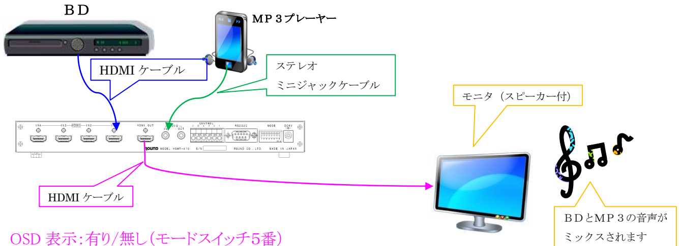
図2:HDMI出力とアナログ音声出力の両方を接続してHDMIモニタ(スピーカー付)に接続した場合。
