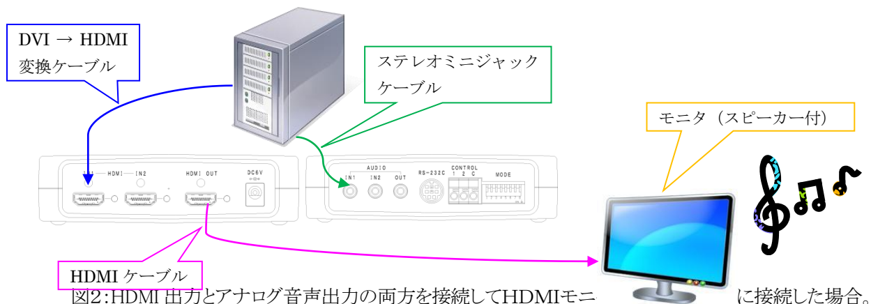
図1:DVI出力/アナログ音声出力のPCをHDMIモニタ(スピーカー付)に接続した場合。
