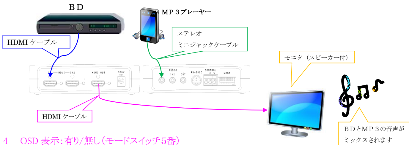
図2:HDMI出力とアナログ音声出力の両方を接続してHDMIモニタに接続した場合。
